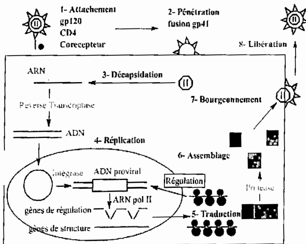
Figure 2 : cycle de réplcation des VIH in : Rothe M, Israël N, Barré SF. Med 1996 [22]
